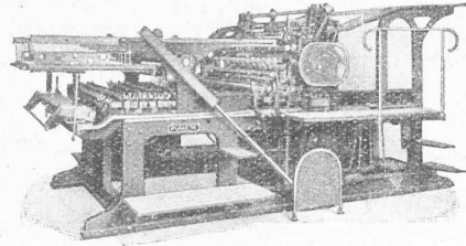
Bildo de „Planeta“, rapidpresmaŝino kun duturna cilindro
