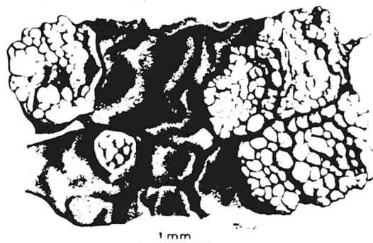
Fig. 48 - Makuloformaj ( Pertusaria amara ).
