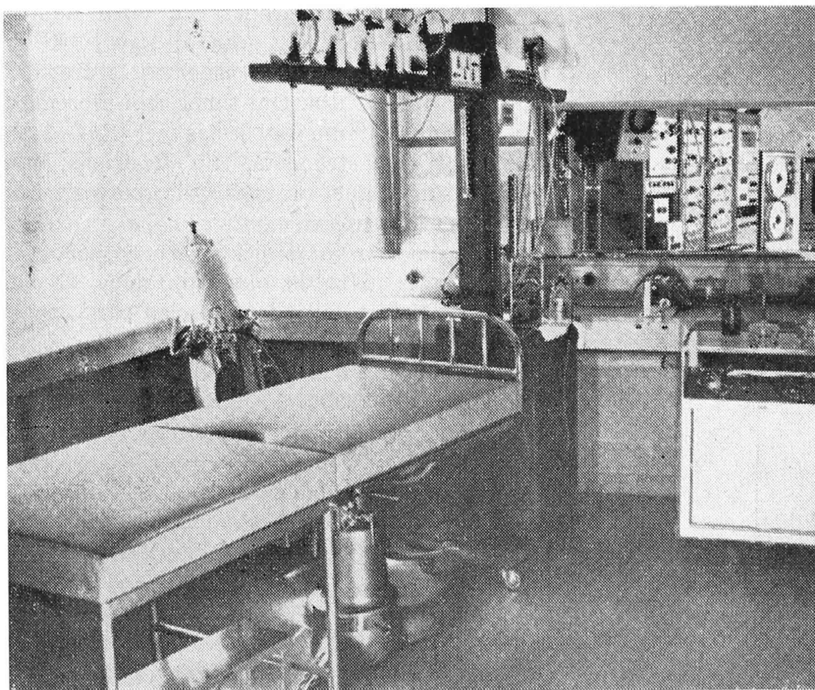
Akuŝĉambro, kie la akuŝantinoj estas flegataj per la elektrona registrado de la amnia tensio, korbata frekvenco de la feto, arteria tensio, vejna tensio, ktp. Tra la fenestro en la fono oni vidas la elektronajn aparatojn utiligatajn por la koncernaj fiziologiaj registradoj en ĉiu akuŝo.
