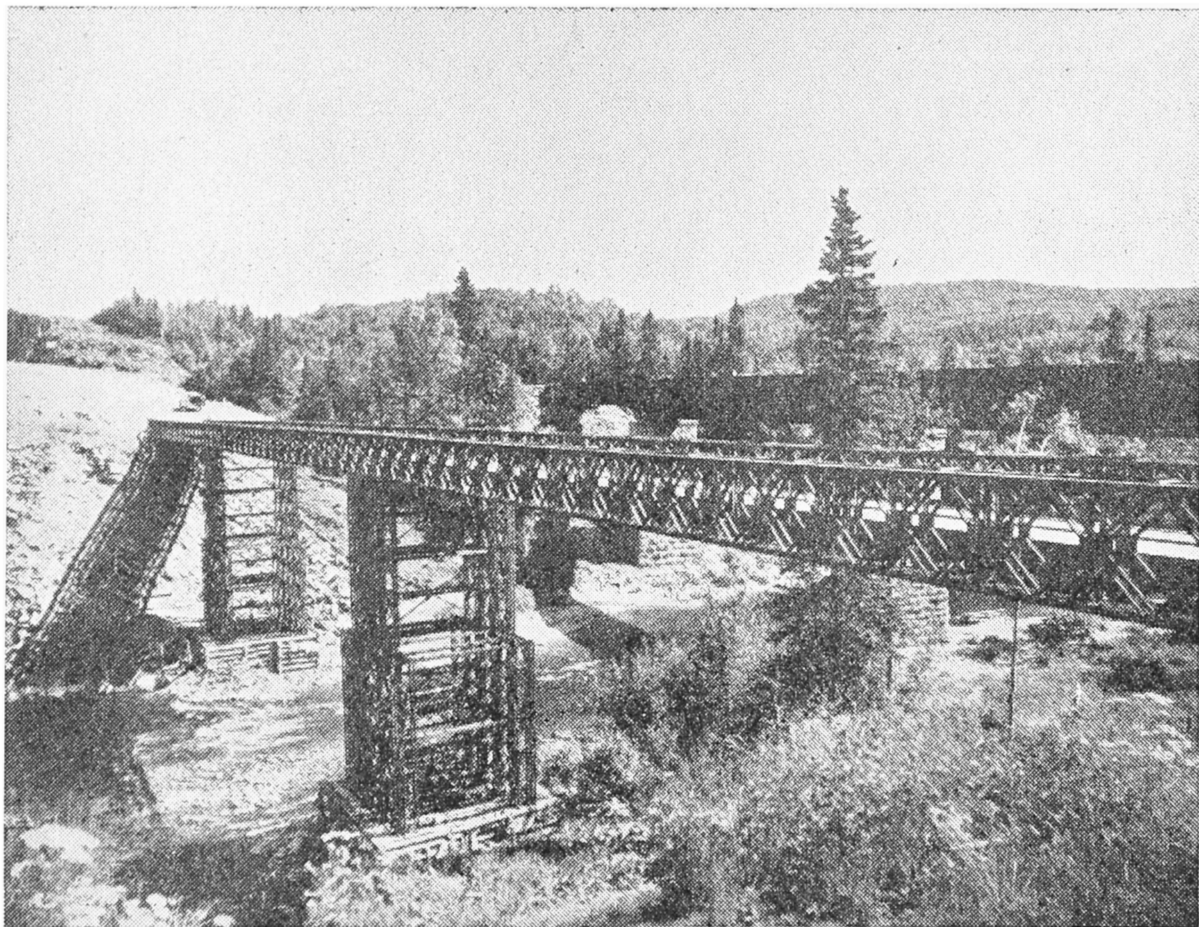
Bailey Ponto super Rivero Steel, Ontario, Kanado (Laŭ afabla permeso de Dept. of Highways, Registaro de Ontario) (Vidu paĝon 299)
