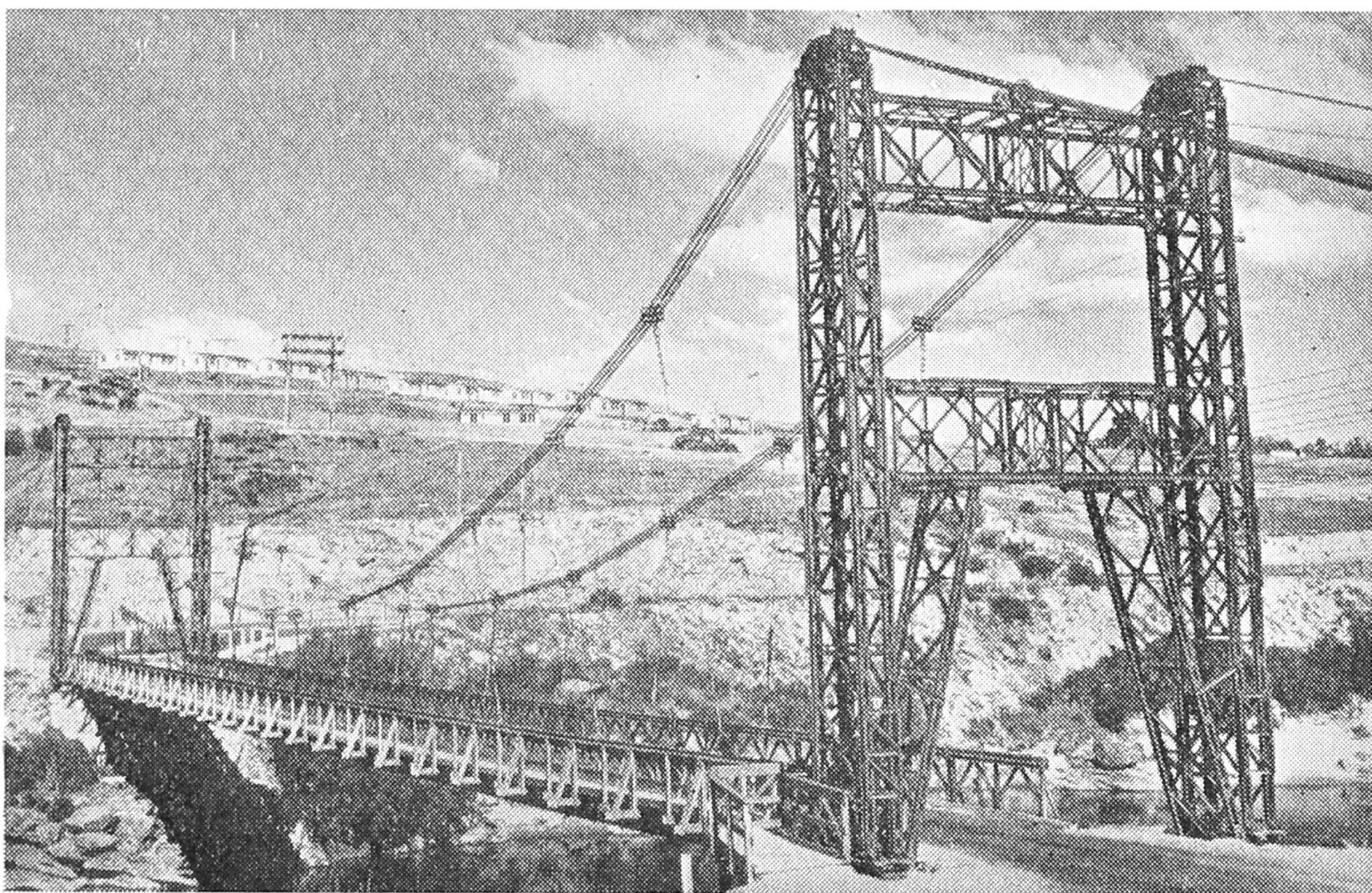
Bailey Ponto super Rivero Clutha, Nov-Zelando
