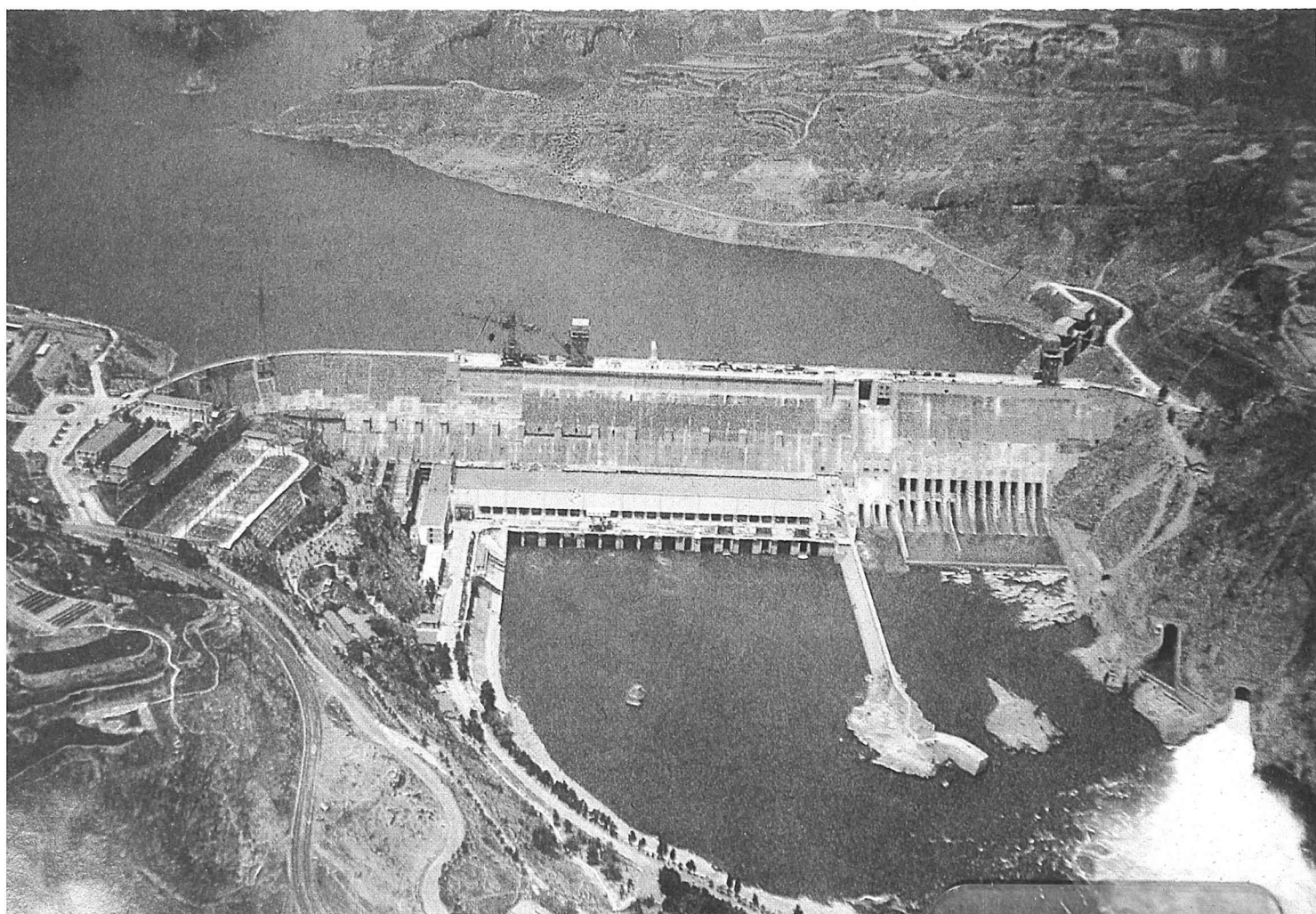
Akvomastruma konstruo en la maisupra parto de la Flava Rivero
