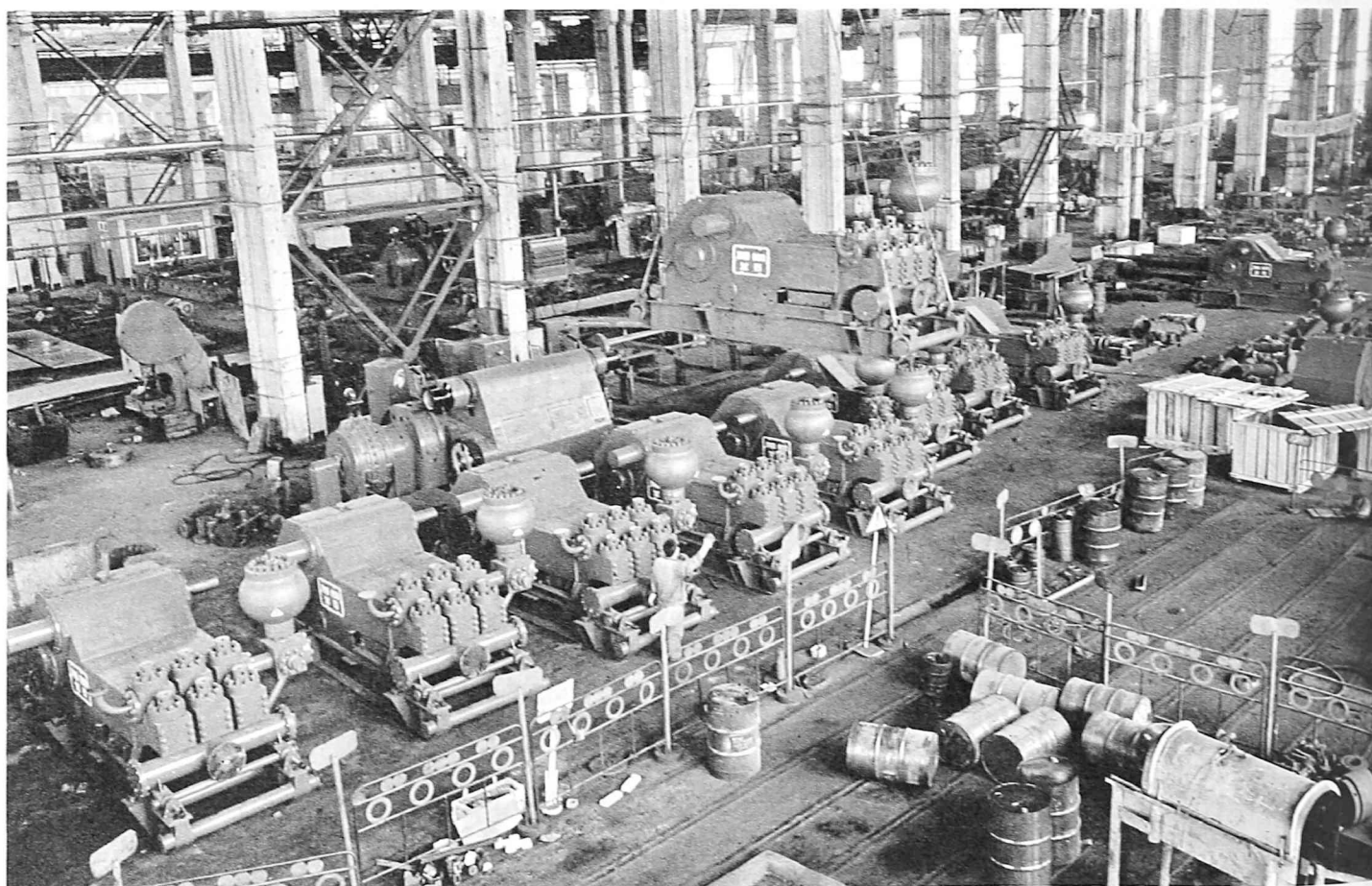
Ŝlim-pumpiloj produktitaj de fabriko de petrol-kemiaj maŝinoj
