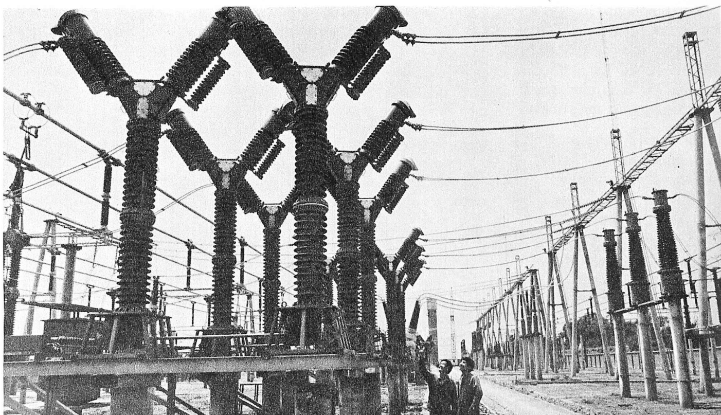
Elektra lineo de 500 kilovoltoj
