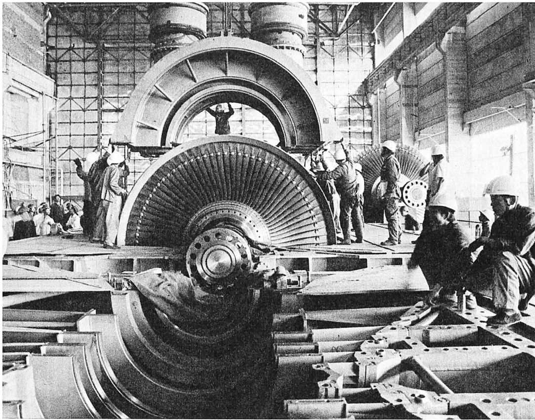
Vaporturbinaj generatoroj ĉiu kun kapacito de 600 mil kilovattoj en streĉa muntado en la Interna Mongolio
