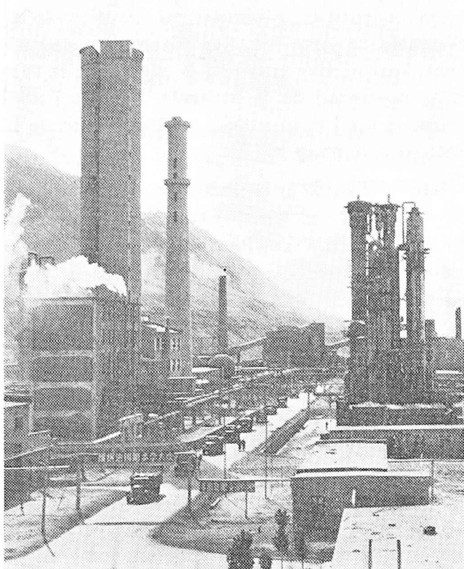
Nova Kemisterka Fabriko de Vulašan kun enlande faritaj ekipaĵoj
