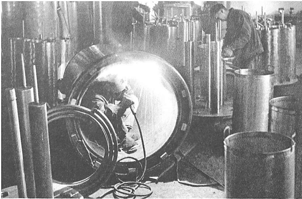
Alttemperaturaj kaj altpremaj tinktur-maŝi- noj pogrande produkta- taj de brigada agrikul- turila fabriko
