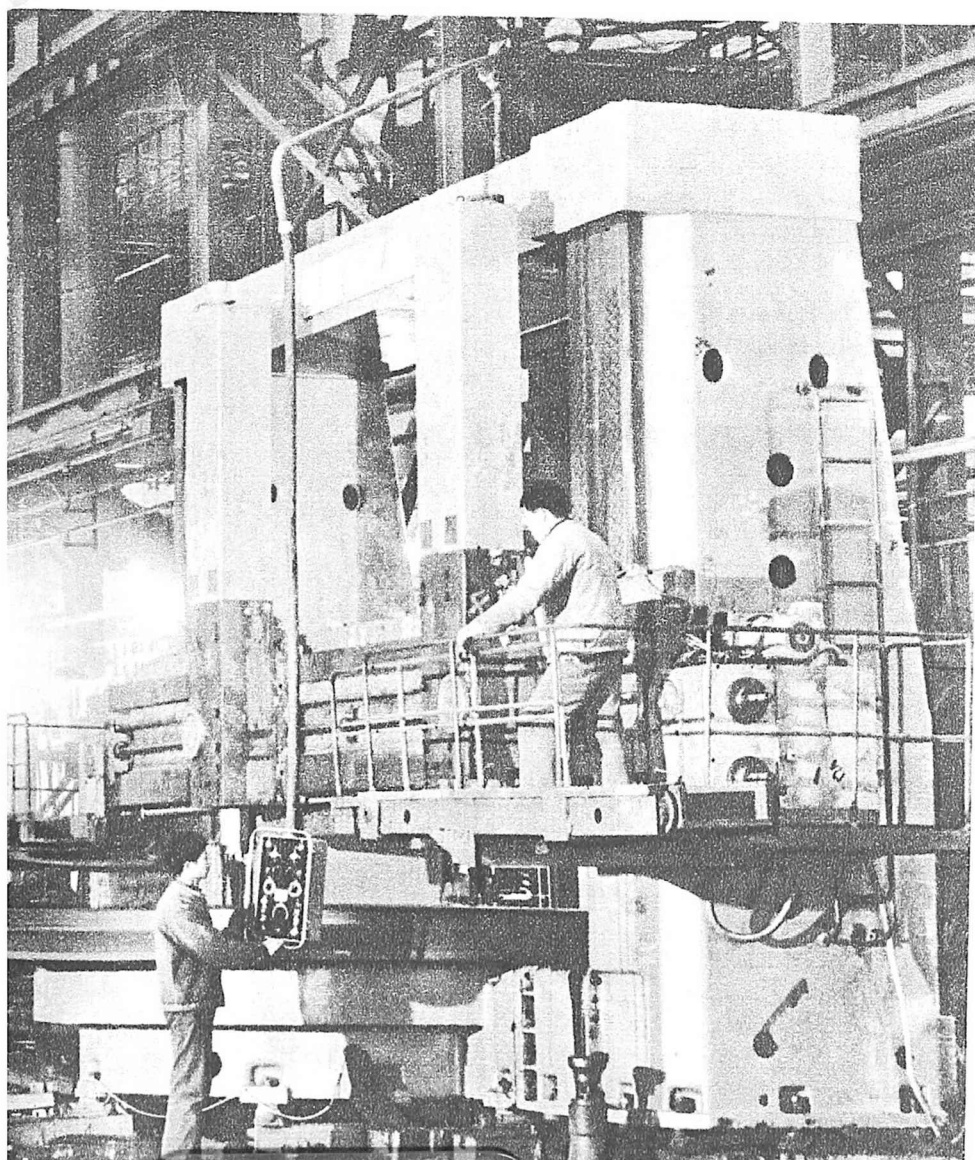
Novaj ilmaŝinoj produktitaj de la Vuhan-a Pezilmaŝina Fabriko
