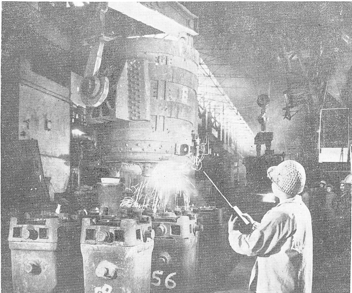
Muldado per teledirekta aparato projektita kaj farita de laboristoj mem
