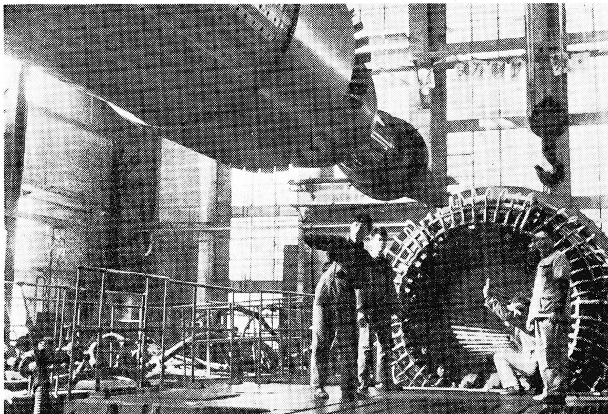
Generato kun interne farita duobla akva malvarmigo en muntado
