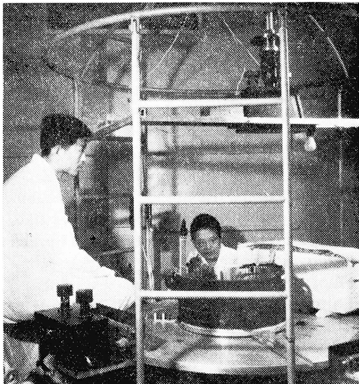
Laborantoj de fizika instituto faras simuladan eksperimenton pri la influo de la varmigo de Kinghaj-Tibeta Altebenajo al ĝenerala cirkulado de la atmosfero en la Orienta Azio en somero.
