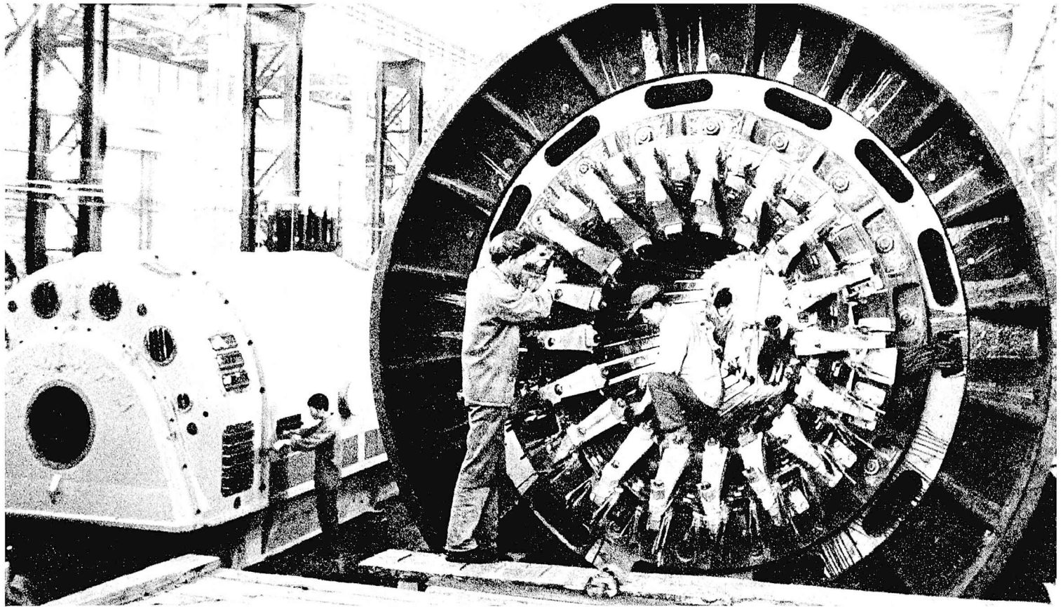
La laboristoj de la Hudong-a Ŝipkonstrua Fabriko mem fabrikis grandtipan tornomaŝinon, kiu povas unufoje fini prilaboradon de kranka instalaĵo de dizelo kun 12,000 ĉevalpovoj. Tio faciligis la pezan prilaboron.
