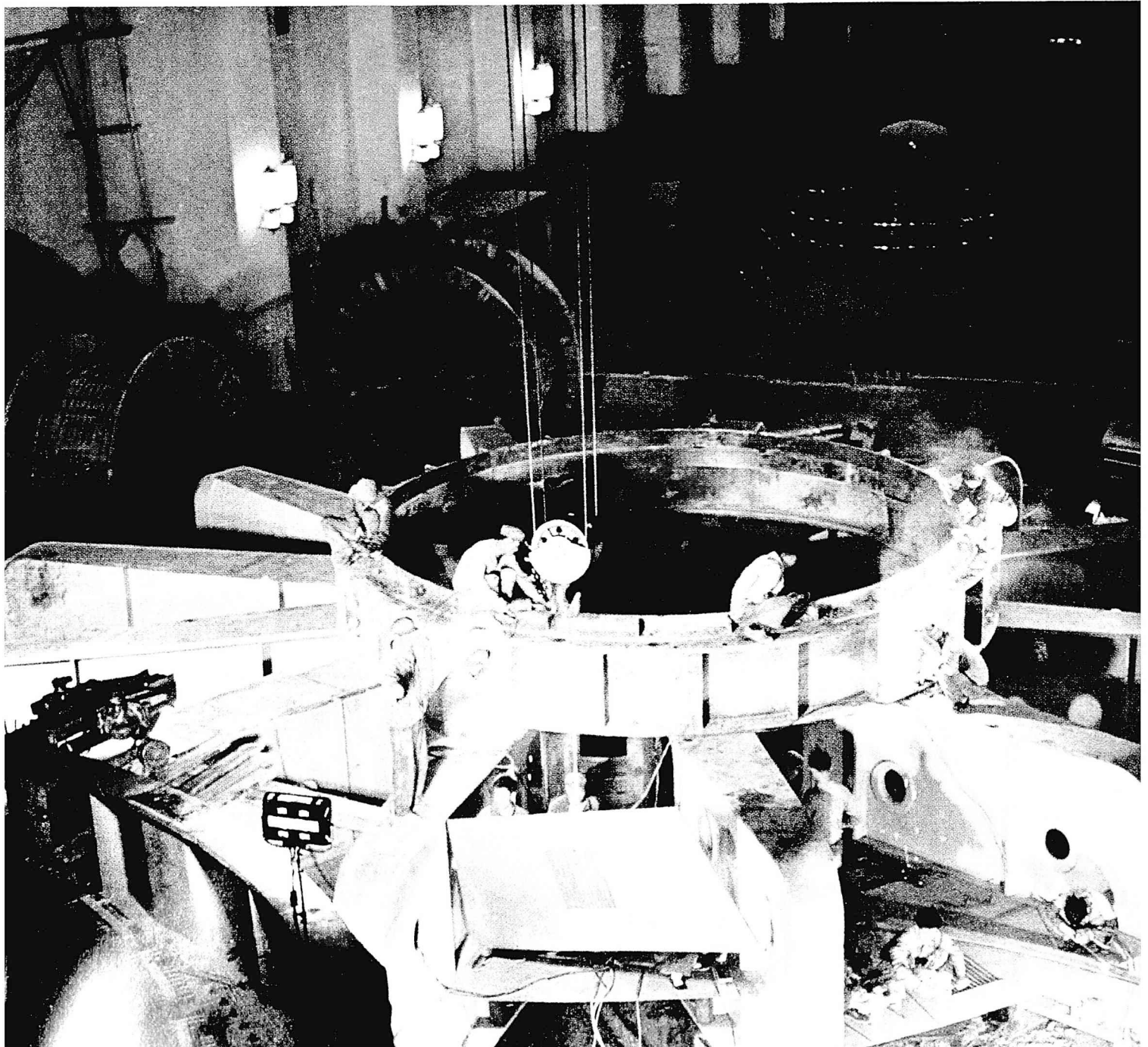
Instali generatoran kompleton
