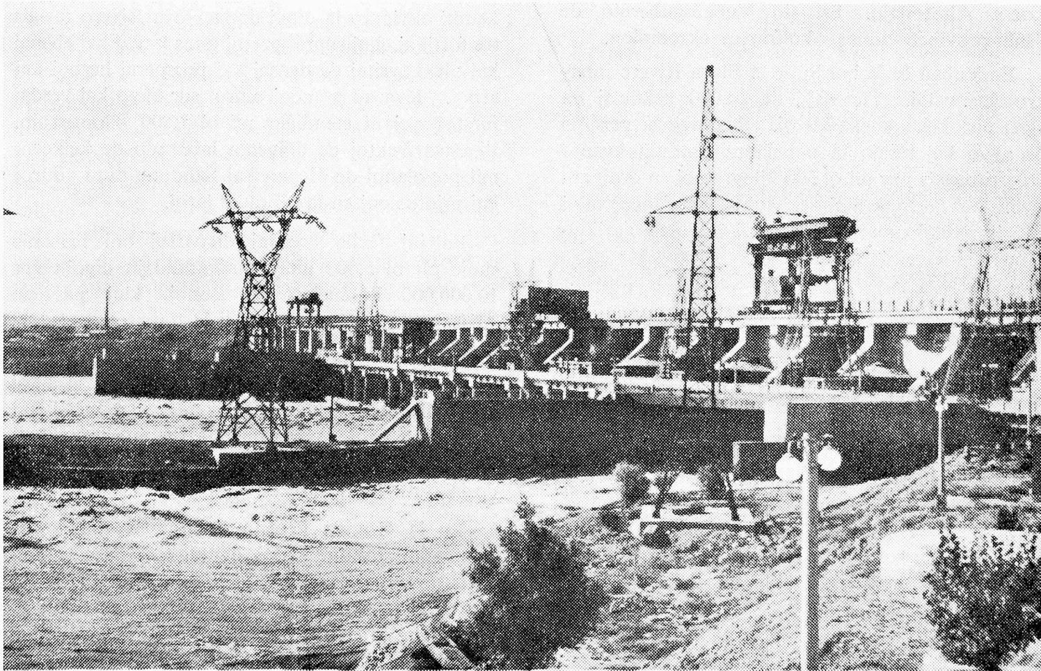
Angulo de la pivota akvoutiliga konstruaĵo Kingtonghia sur la Flava Rivero
