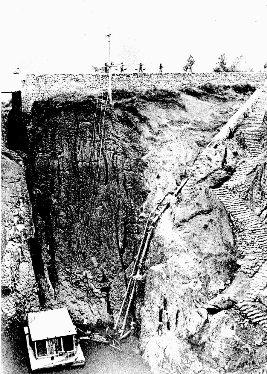
Pumpi subteran akvon per pumpilo sur cementa boato fiksita ĉe la malkaŝita fenestro de subtera rivero
