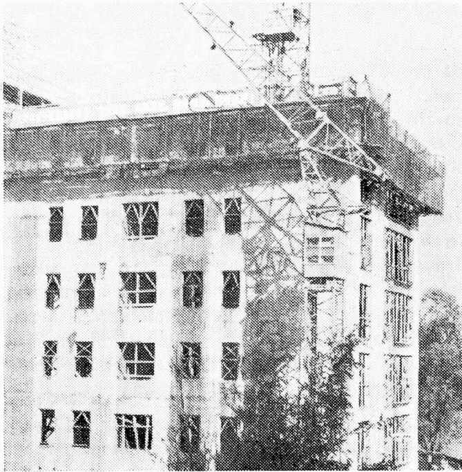
Glit-forma tabulo estas leviĝanta.
