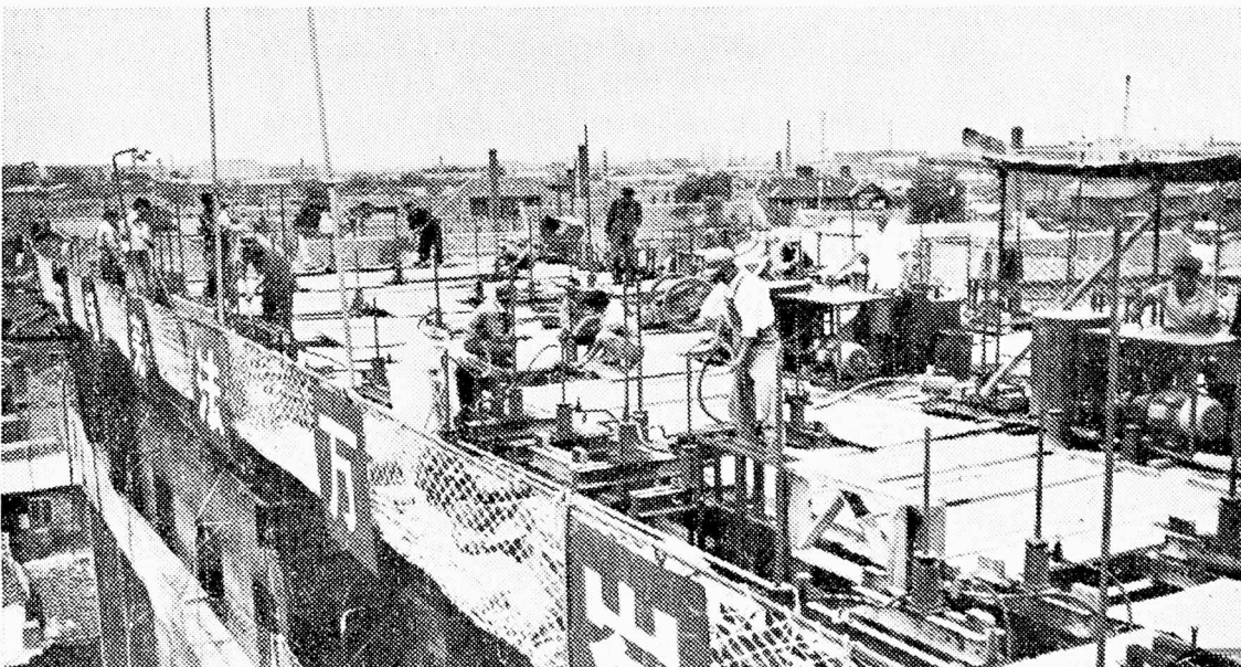
Ŝenĵang-aj konstruaj laboristoj konstruas etaĝan domon aplikante glit-forman konstruan teknikon.
