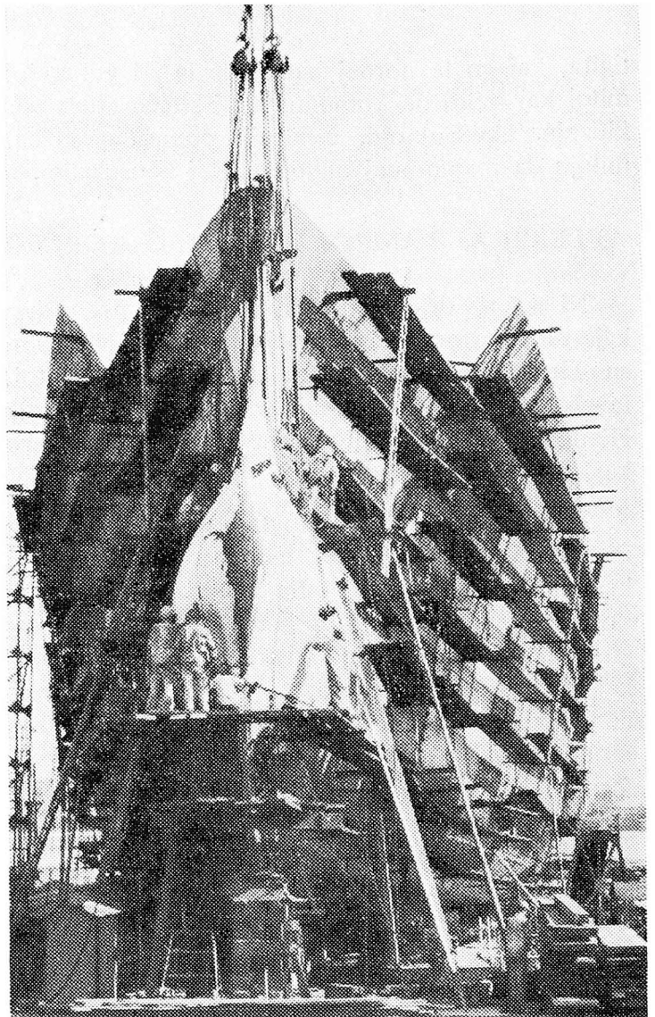
Globforma steveno de dekmil-tonela ŝipo en muntado
