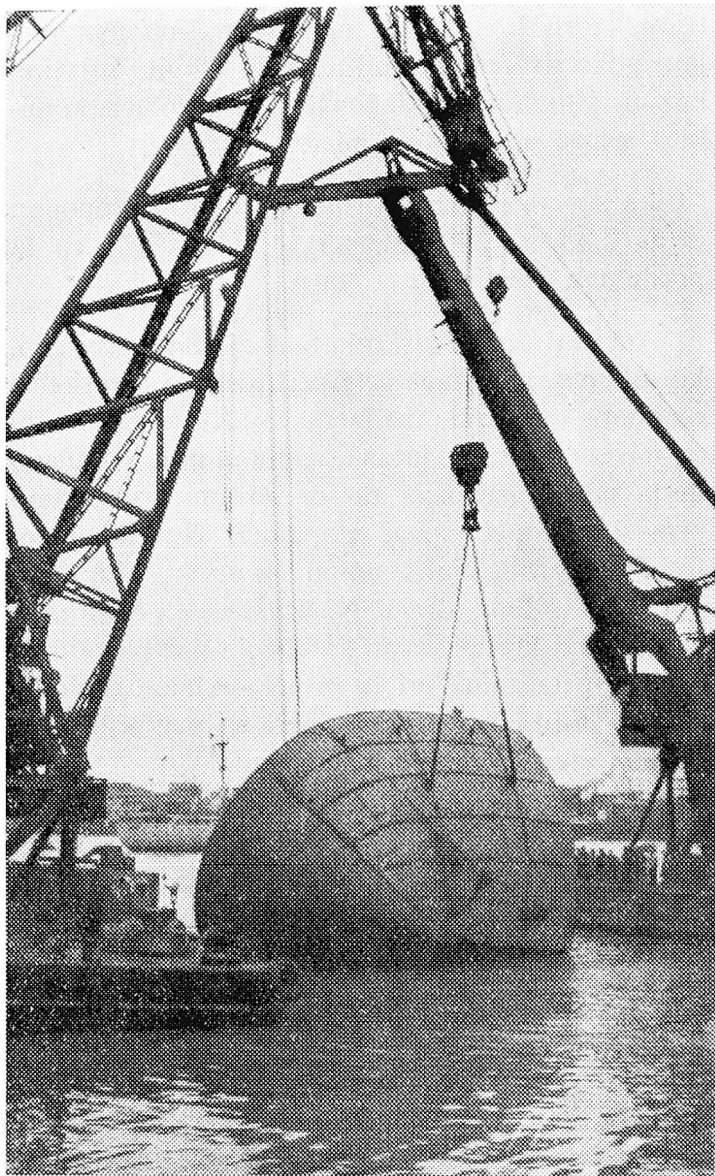
Poŭpo 107 tunojn peza en surakva renversado
