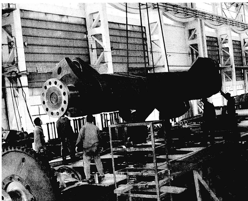
Muntado de krankŝafto al 10,000-ĉevalpova dizelo
