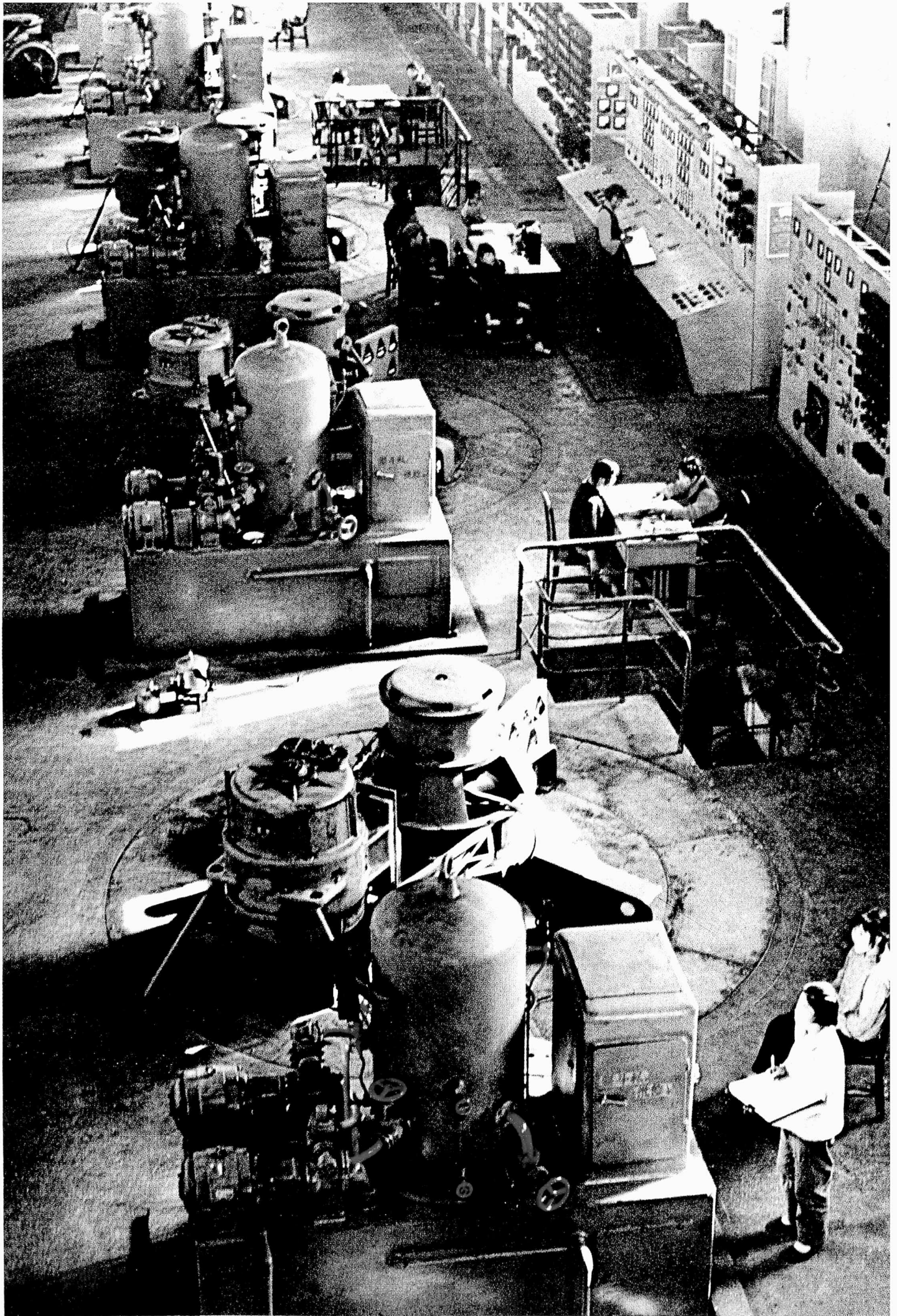
La hidroelektra centralo Nagin de Lasao
