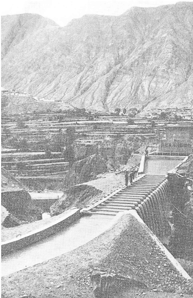
Hidroelektra stacio Gulandi de Kinghaj-provinco
