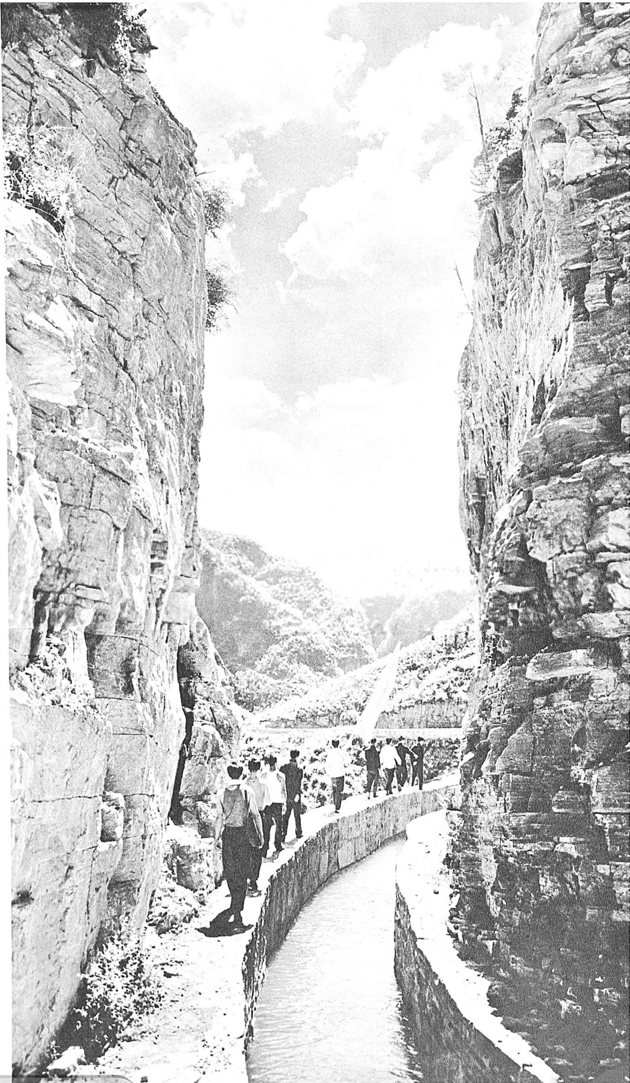
La akvokonduka kanalo sin direk- tas al la elektra stacio.
