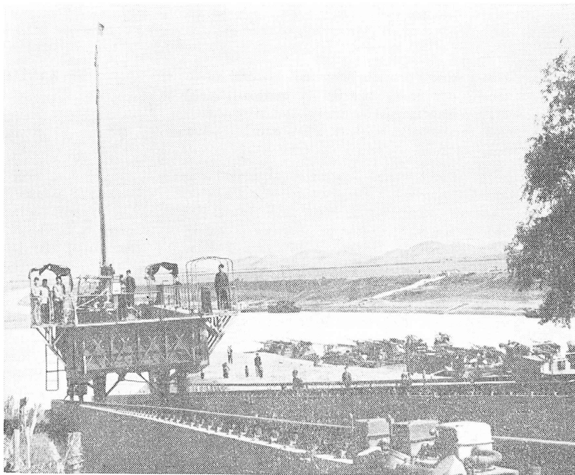
Elektra ŝiptransportilo de la Granda Kluzo de Fejsuj-rivero portas ŝipon trans digon.
