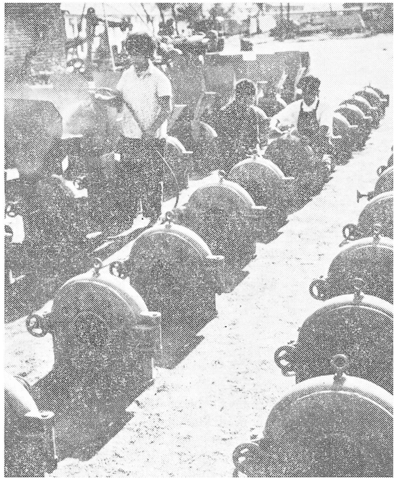
Altrapidecaj dispecigaj maŝinoj produktitaj de la gubernia fabriko de agrikulturaj instrumentoj por la kamparo
