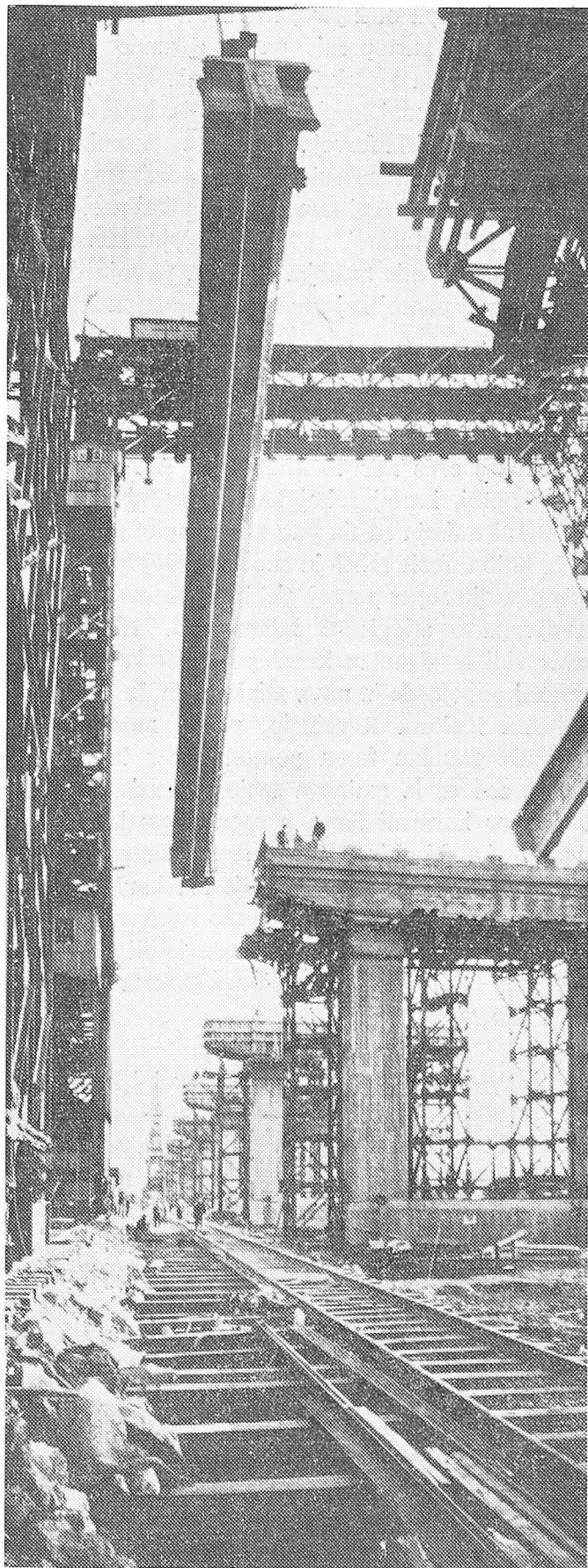
La Nankina pontego super Jangzi-rivero en konstruado
