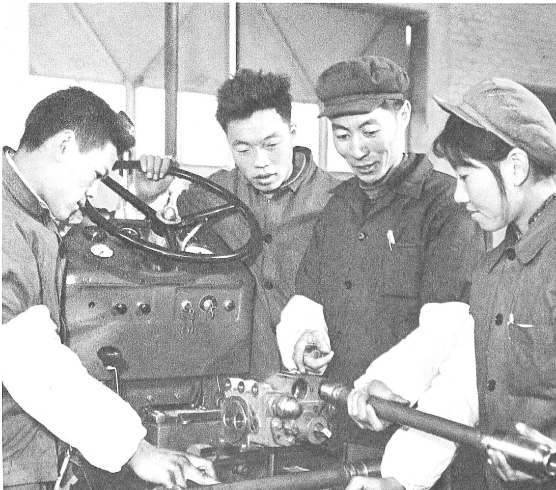
Laboristoj de la Fabriko de Hidrostatikaj Elementoj de Ĉanggi muntas hidrostatikan traktoron kun 40 ĉevalpovo.
