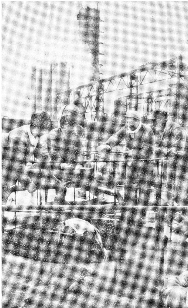
Laboristoj ŝanĝis venenan akvon en sterkan akvon utilan al kreskado de agrikulturaj plantoj forigante fenolon per mikroboj.
