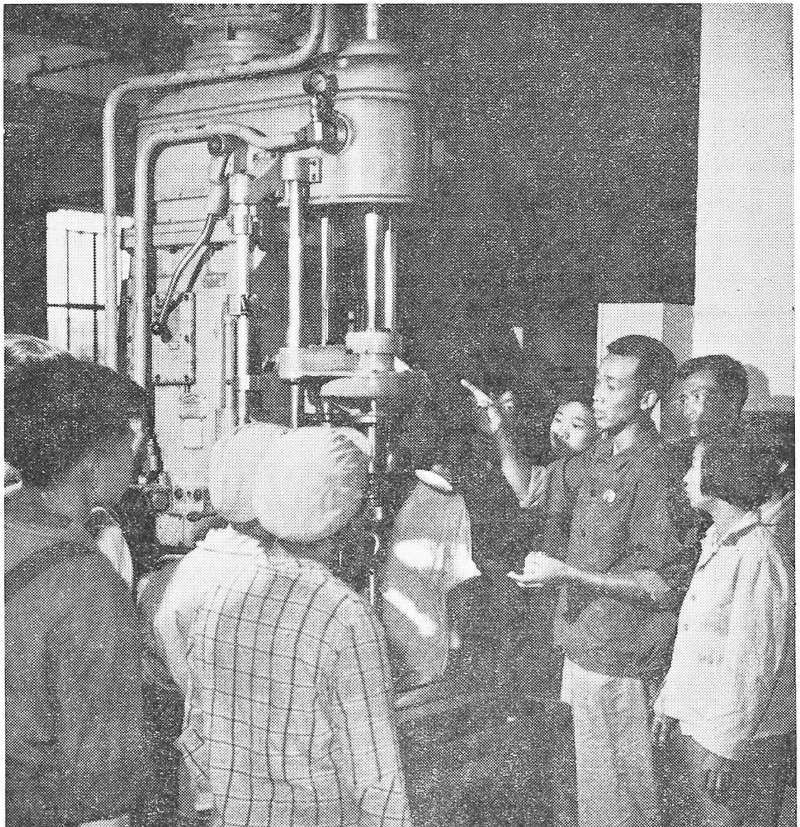
La laborista studento kun praktika sperto riparis importitan maŝinon, kiu estis forlasita en la mekanika fakultato jam 13 jarojn.
