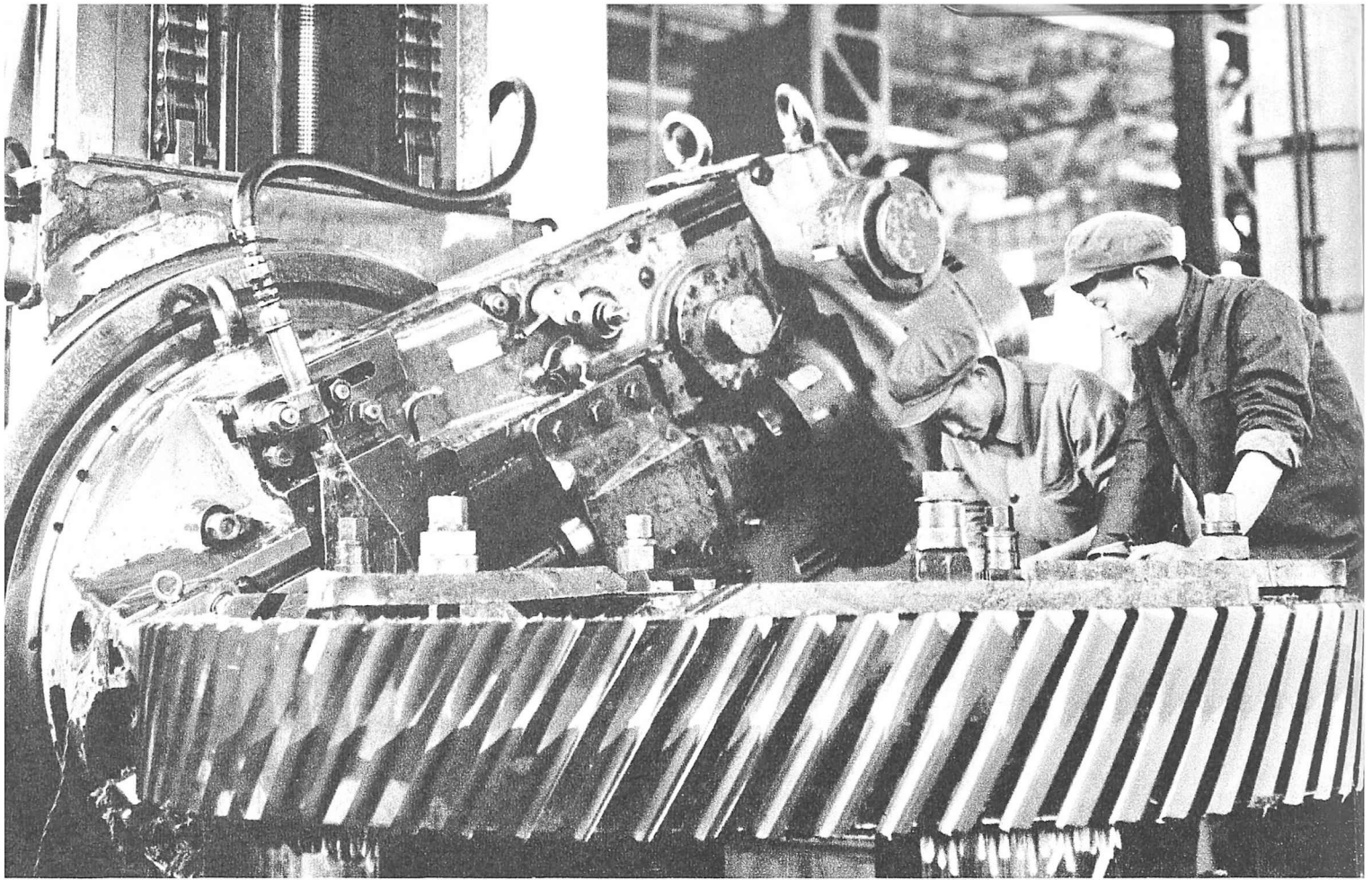
Laboristoj de la Nanŝan-a Fer-minejo de la Maanŝan-a Fera kaj Ŝtala Kompanio sukcesis mem fari ekipaĵon por ercolavado.
