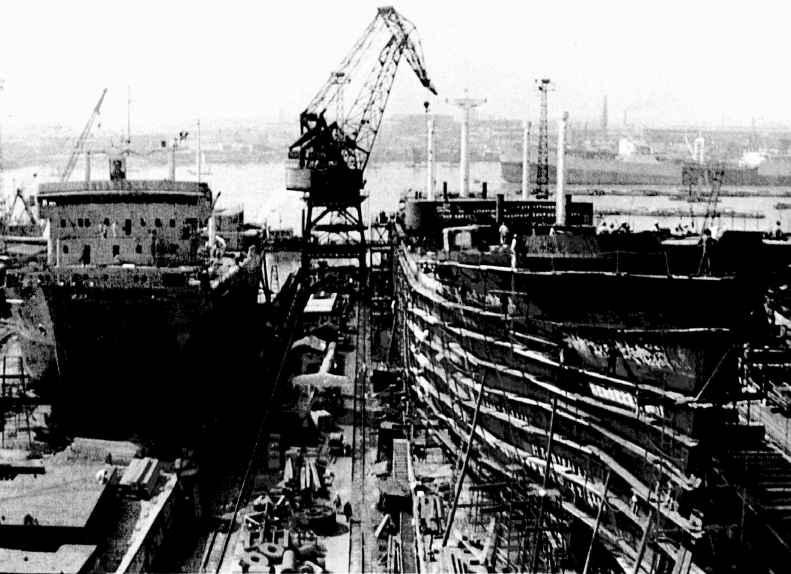
La 10,000-tonelaj ŝipoj "Juejang" kaj "Hianfeng" estas en konstruado.
