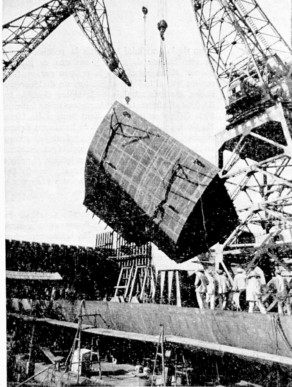
Laboristoj kreis la metodon "turni en la aero", kaj per tio multe altigis la laborefikon en muntado.
