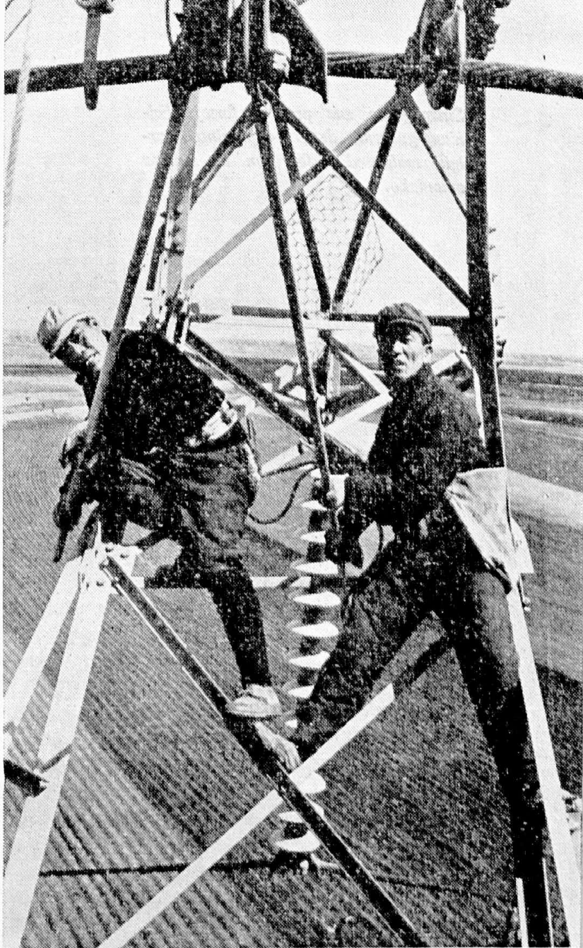
Ĝeng Dajju (la dekstra), inĝeniero de la Anŝan-a Elektro-administrejo kune kun laboristo sukcese faris laboron sur linio de 220,000-volta tensio sen interrompo de kurento.
