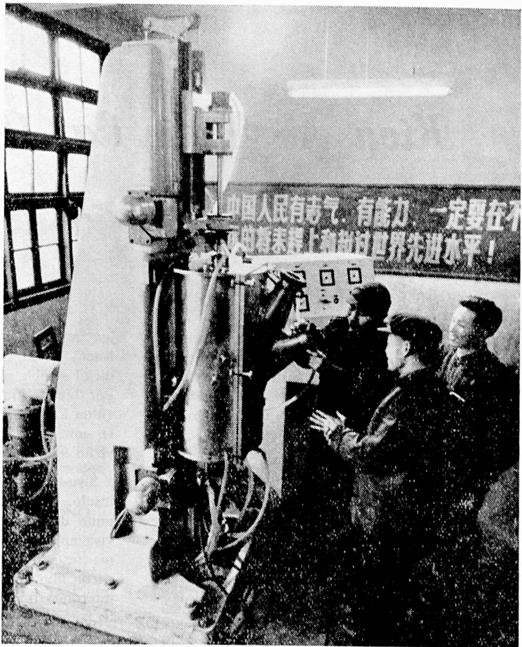
Ĉinstila forno por kreskigo de solkristalo
