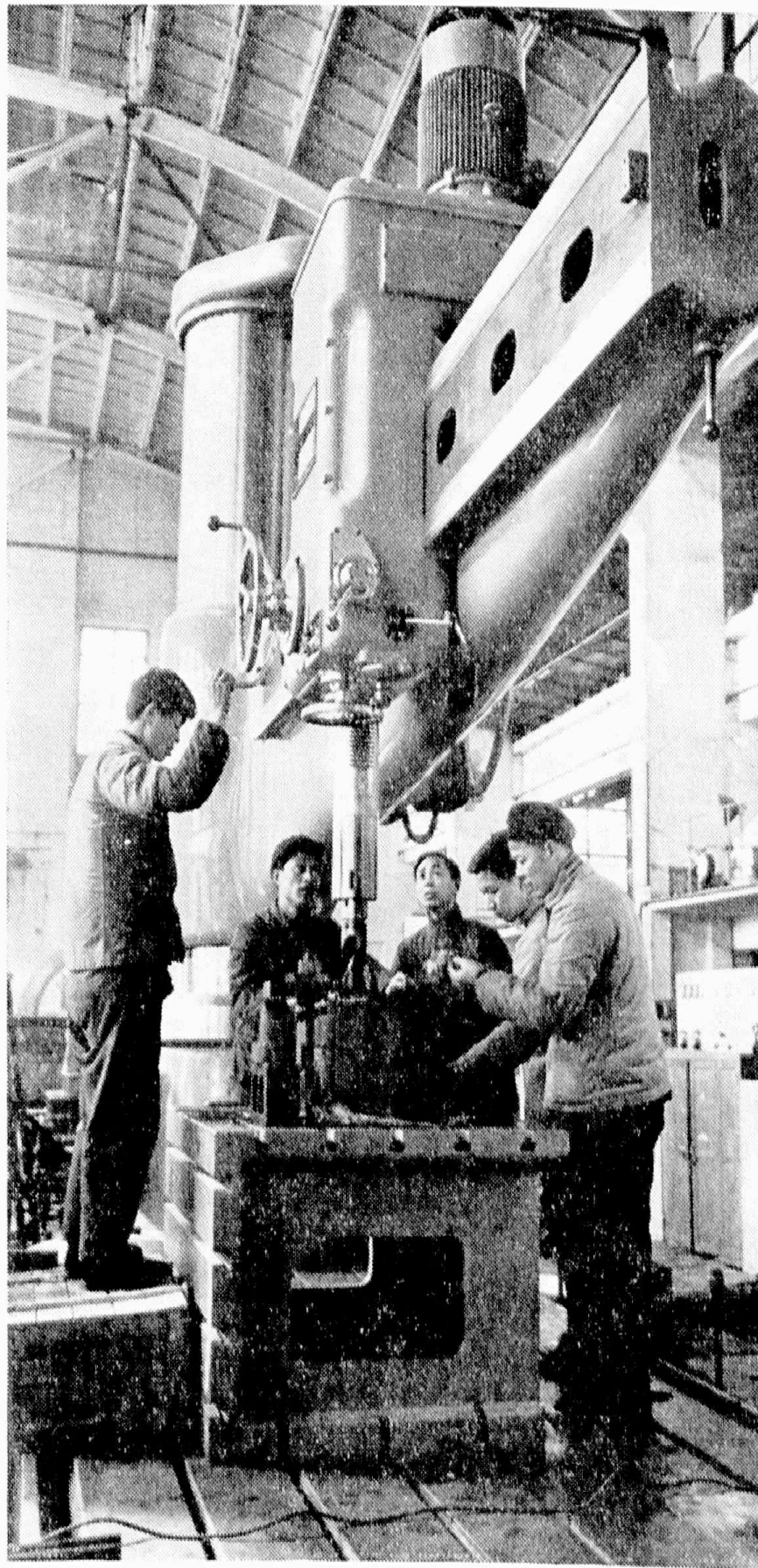
La revoluciaj laboristoj kaj oficistoj en la sfero de la meĥanika elektra industrio de Ŝanhajo projektis kaj provfaris gigantan radio-drilmaŝinon. Peza je ĉ. 45 tunoj kun maksimuma drilkalibro de 120 mm. kaj progresinta strukturo ĝi estas plejparte movata elektre kaj hidraŭlike. Ĝi estas simple kaj facile manipulebla, funkcias stabile kaj multe konformas al la bezono de prilaboro de grandaj maŝinpecoj.
