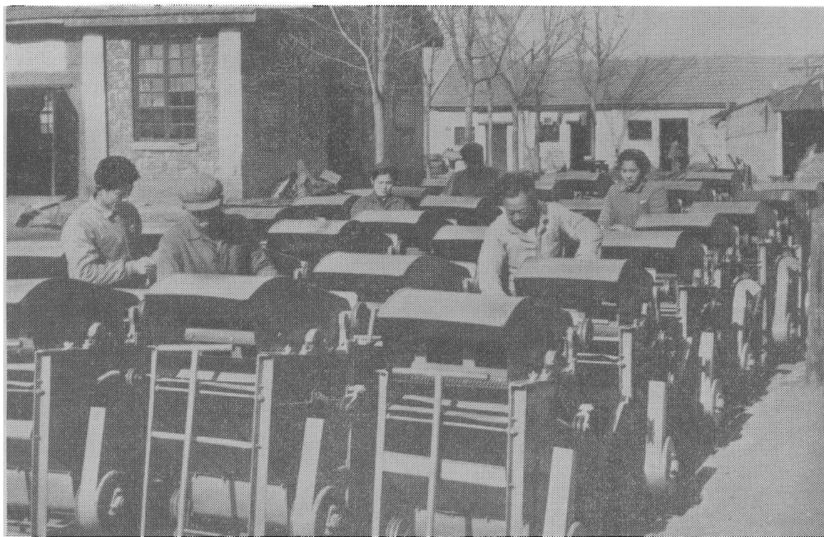
La maŝinfabrika de Tanghe-gubernio, Henan-provinco, sukcesis fari draŝan kaj tranĉan maŝinon "tipo 45", kiu povas draŝi grenajn plantojn kaj tranĉi fojnon.
