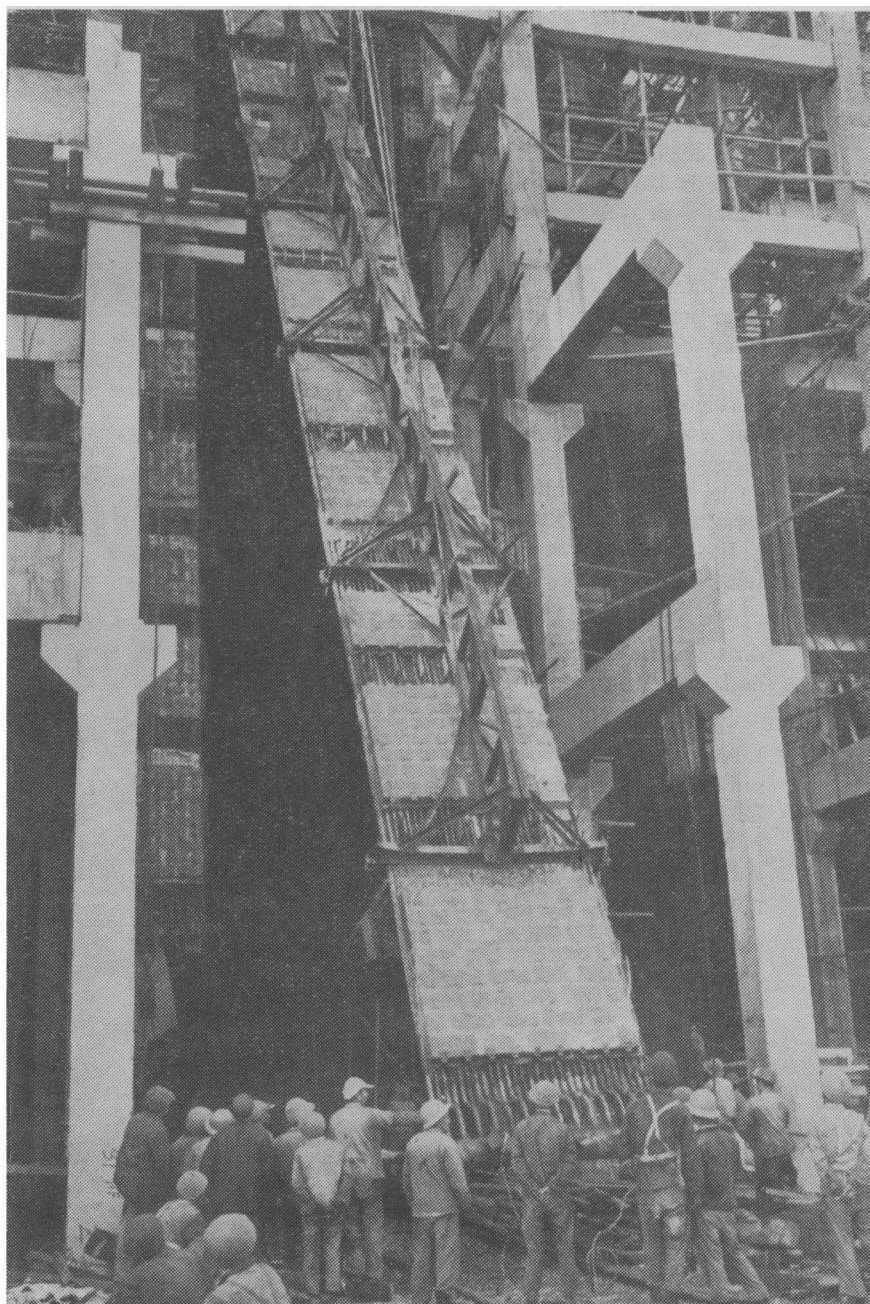
La muntistoj levas kaj fiksas akvomalvarmigan muron al la kaldronego.
