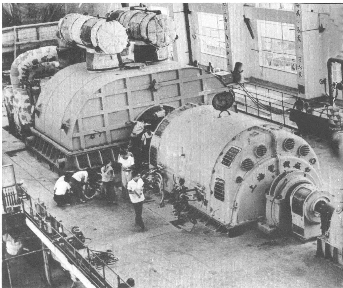
(Supre) La 125,000-kilovata vaporturbina generatora kompleto kun duobla akva interna malvarmigo
