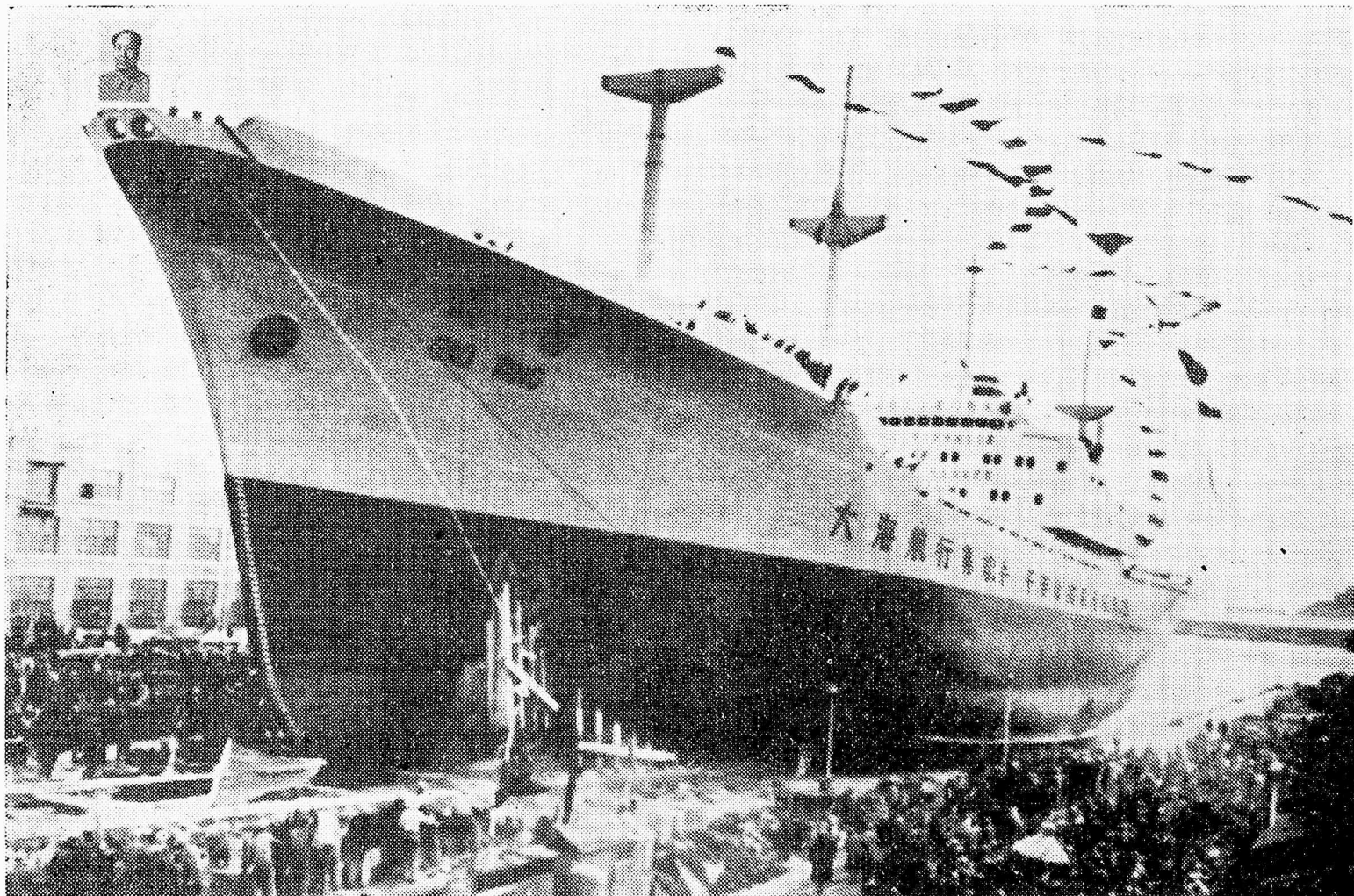
Dekmiltonela oceana ŝipo “Gao Yang”
