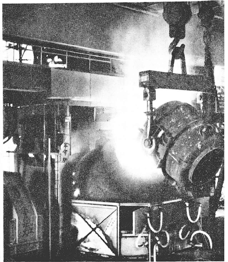
La unua laborejo de aŭtomata konvertil-forno de supra blovado per pura oksigeno en nia lando estas funkcionstruita. Jen laboristoj laboras en manipulejo (maldekstre) por (dekstre) direkti la fornon en fando de ŝtalo.
