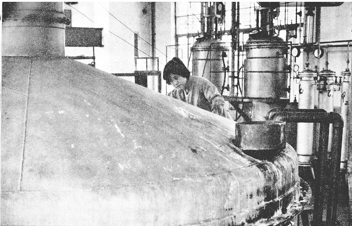
En nia lando oni uzas mikrobojn por liberigi petrolon de parafino kaj tiel produktas atklasan petrolan produkton de malalta solidiĝa punkto. La kvalito multe superis tiun de la samspeca petrolo produkto el eksterlando. Jen la granda fermentujo de la Ŝanhaja Fermenta Fabriko en uzado.
